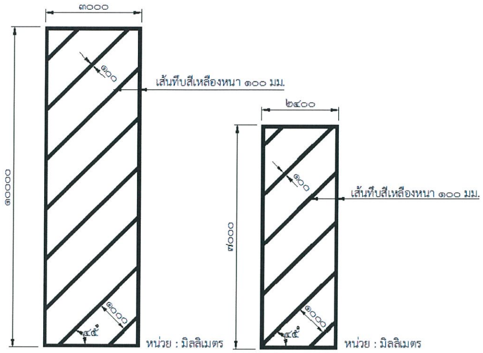
รูปที่ ๓ พื้นสำหรับรถดับเพลิง รูปที่ ๔ พื้นสำหรับรถพยาบาลหรือรถปฏิบัติการฉุกเฉิน
